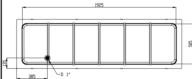
Boven aanzicht
